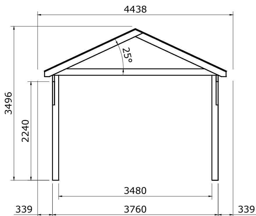
Rechter zijaanzicht
